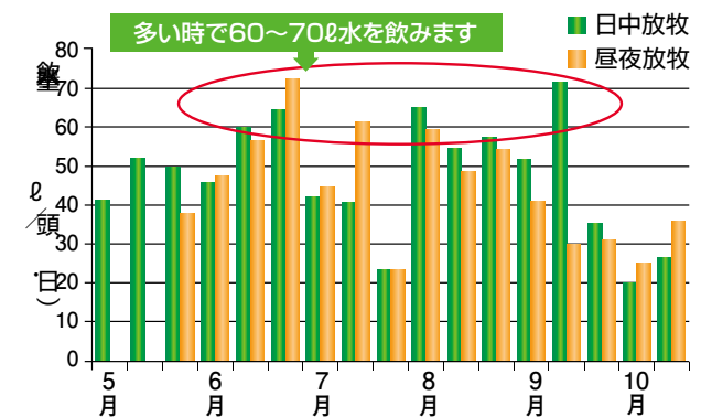
図3 放牧地の飲水量(上川農試天北支場2006)
