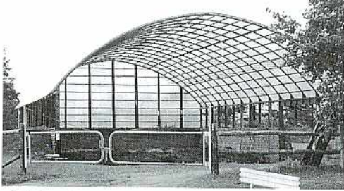
中林牧場（JA中標準） 特徴 ● 敷料の適度な使用 ● 雨水混入防止により堆肥化を可能とする。 ● 圃場の簡易堆肥盤の整備 ● 堆肥の共同散布 ● 設置年・平成6年9月 ● 施設規模・6間×8間（369㎡）
