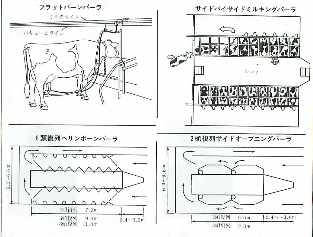
図1. ミルクングパーラの主な種類
